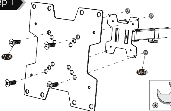
Nut M-B (x4)
